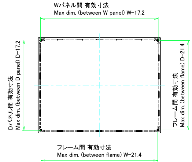
下カバー / Bottom cover
